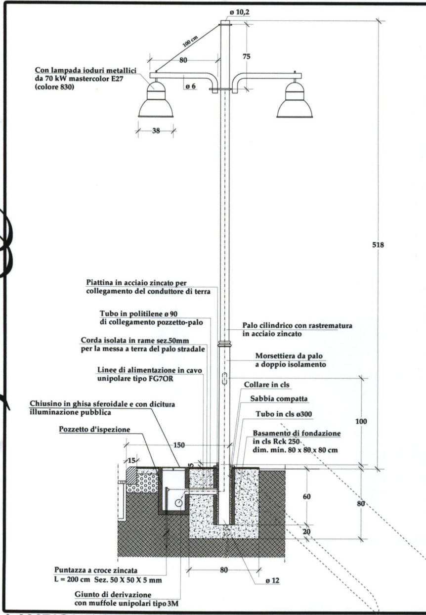
LAMPIONE STRADALE
