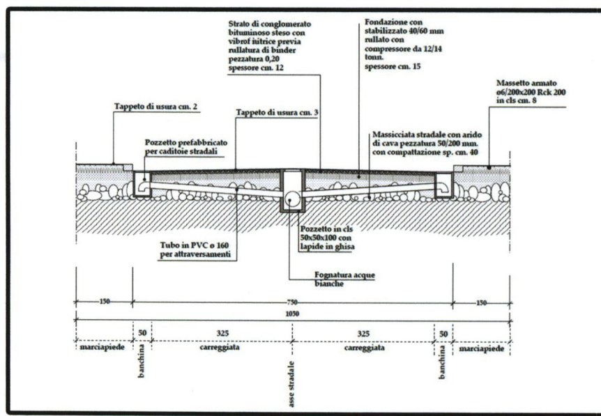
SEZIONE STRADALE
