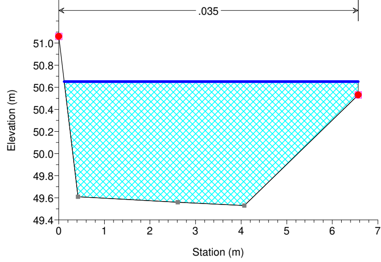
Quarrata_TR200_Tp12h con Stella River = Impialla Reach = Impialla RS = 455.83*
