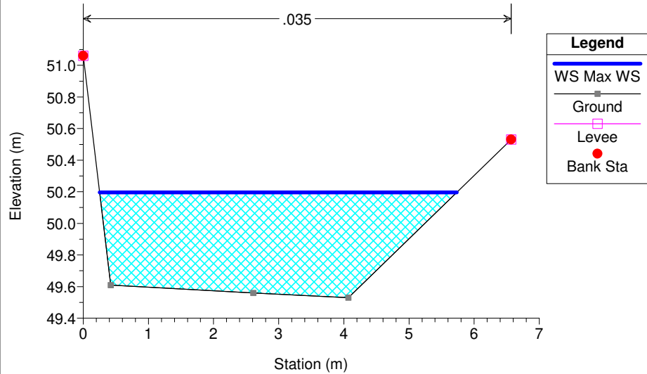
Quarrata_TR200_Tp24h con Stella River = Impialla Reach = Impialla RS = 456.67*
