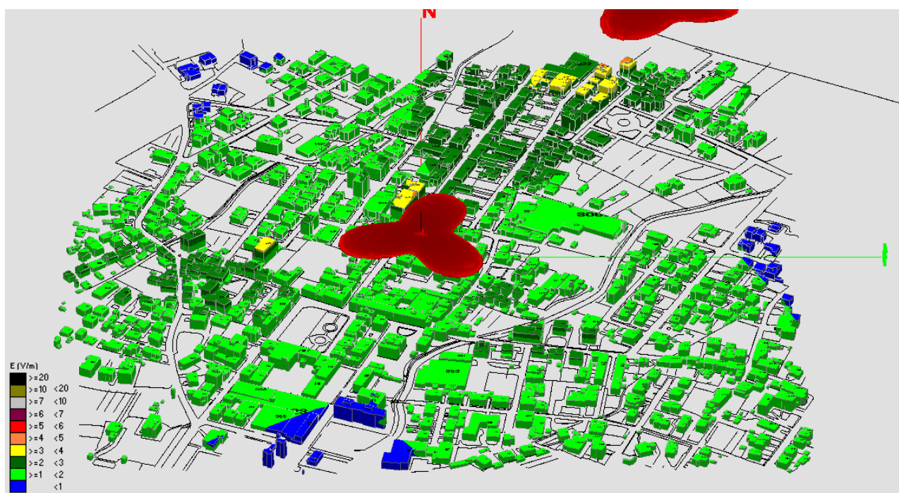
Fig. 16 Impatto elettromagnetico – Zona Via Mazzini – 0°/Nord
