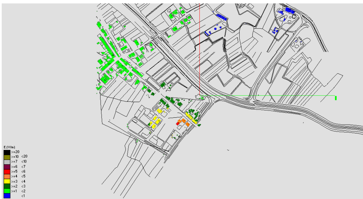
Fig. 27 Impatto elettromagnetico - Zona Depuratore Via SS Pistoiese - conf Carmignano - Vista dall'alto 2
