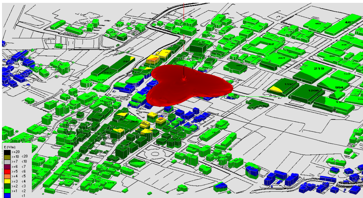
Fig. 13 Impatto elettromagnetico – Zona Centrale TELECOM Via Tiziano – 0°/Nord
