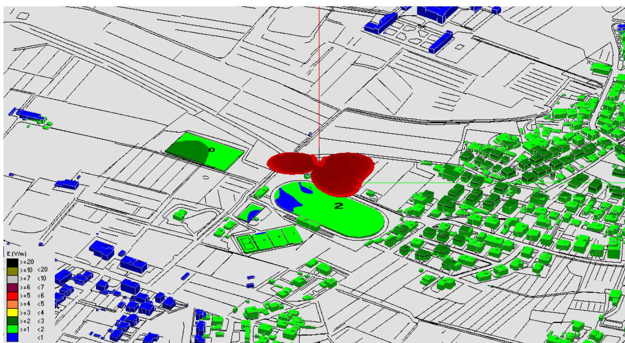
Fig. 19 Impatto elettromagnetico – Zona Stadio Comunale – 0°/Nord
