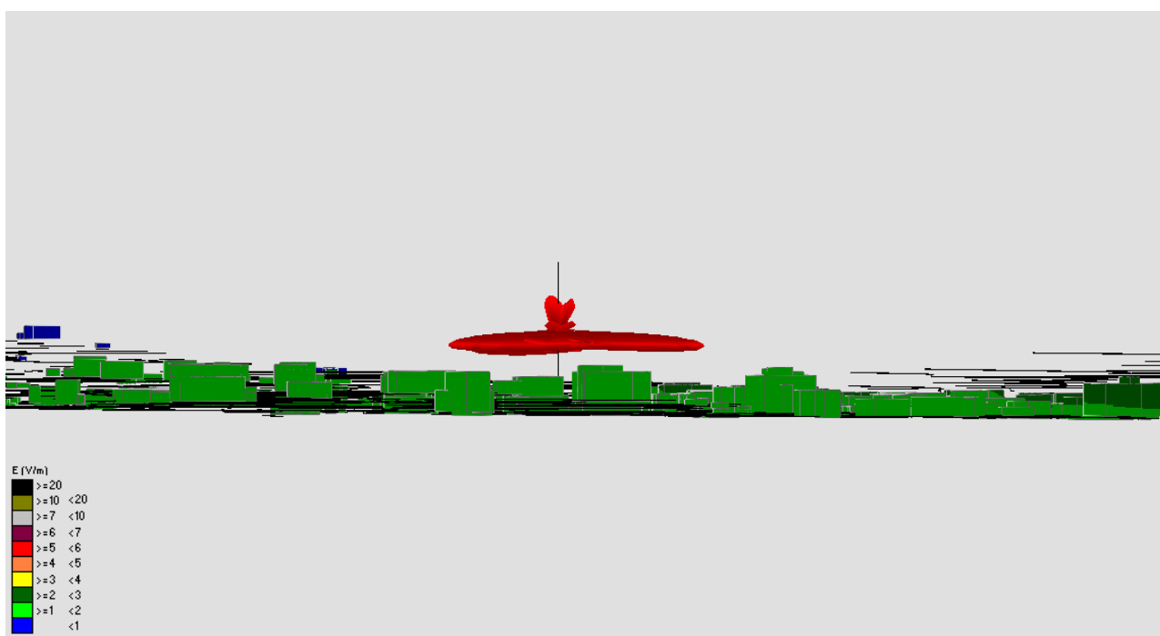
Fig. 21 Impatto elettromagnetico – Zona Stadio Comunale – Vista Laterale
