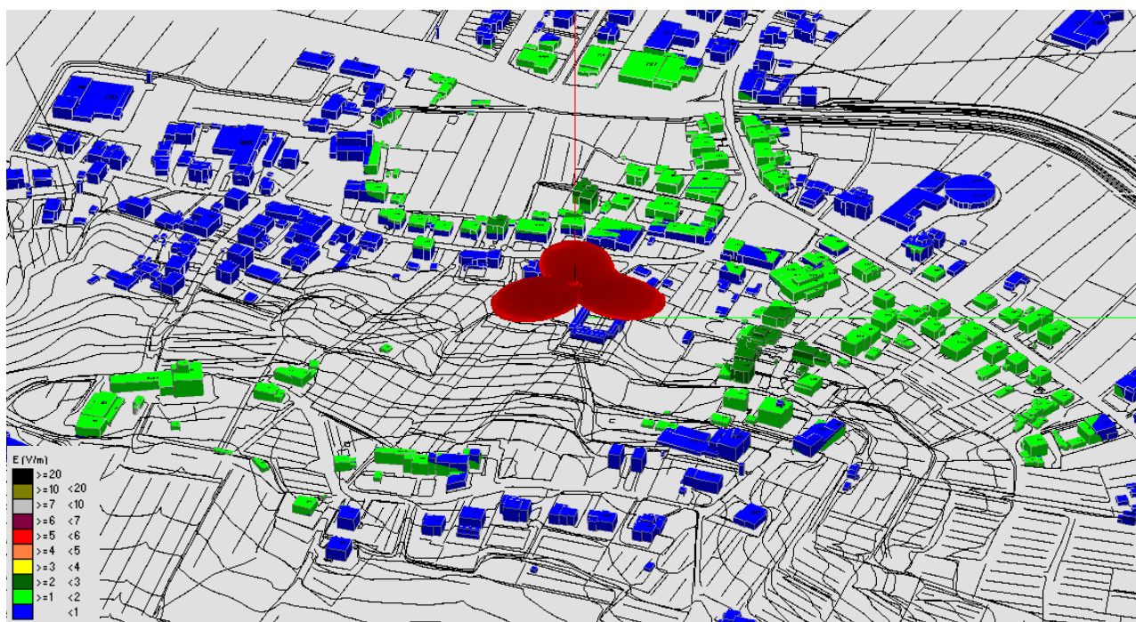
Fig. 4 Impatto elettromagnetico – Zona Cimitero Valenzatico – 0°/Nord
