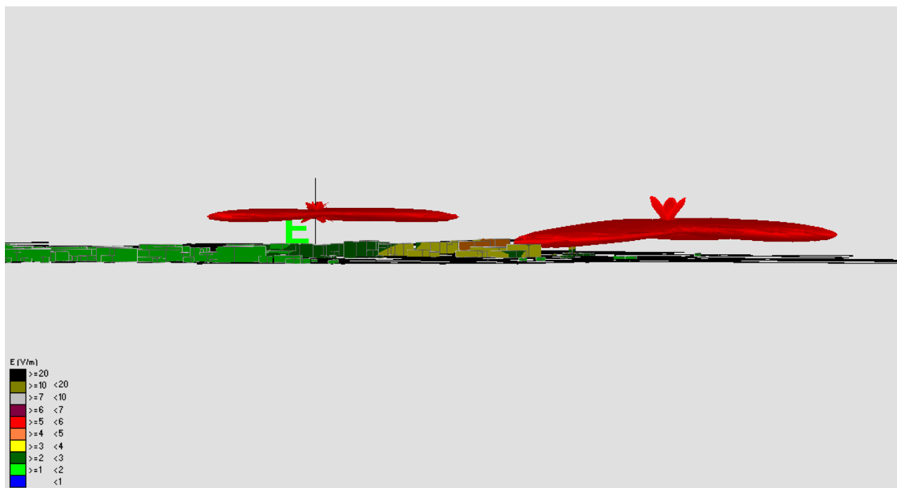
Fig. 28 Impatto elettromagnetico - Zona Depuratore Via SS Pistoiese - conf Carmignano - Vista Laterale
