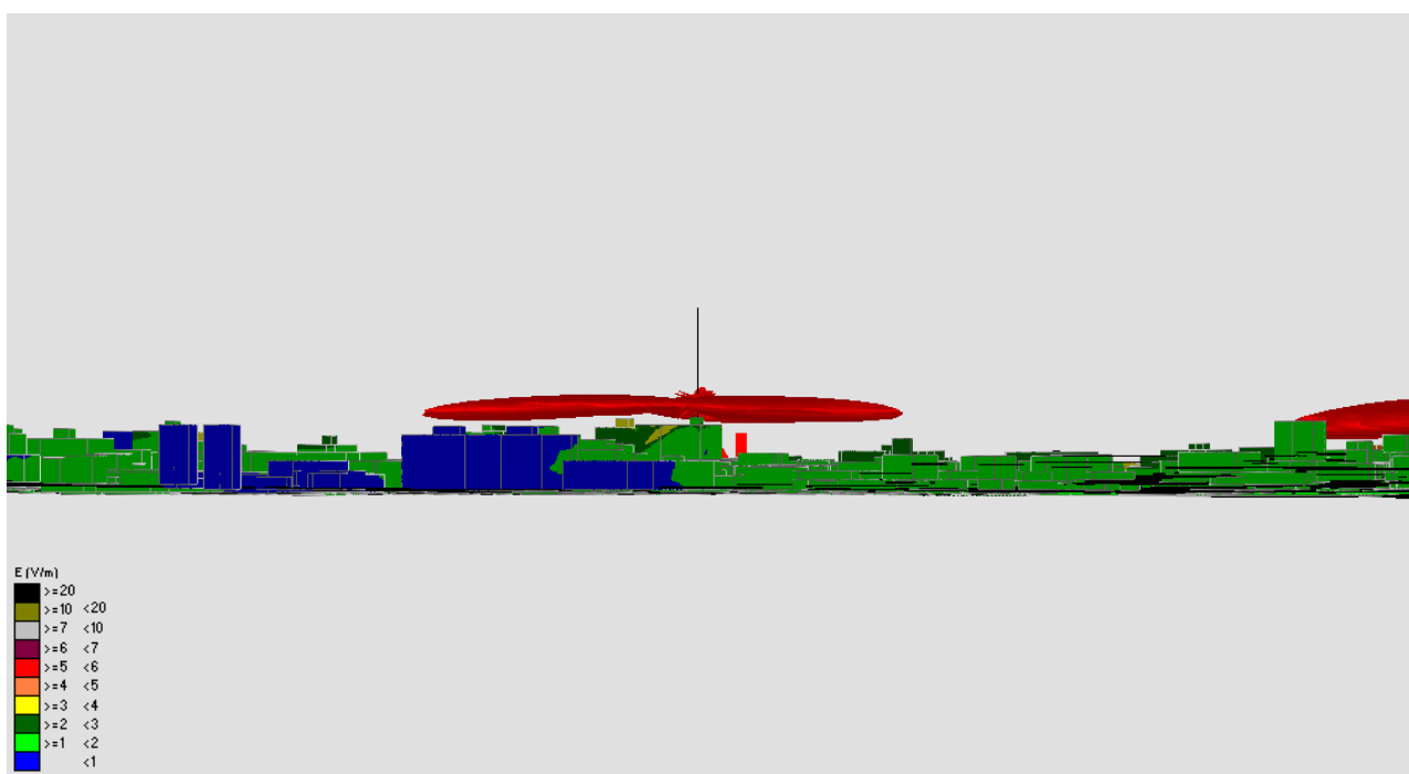
Fig. 18 Impatto elettromagnetico – Zona Via Mazzini – Vista Laterale
