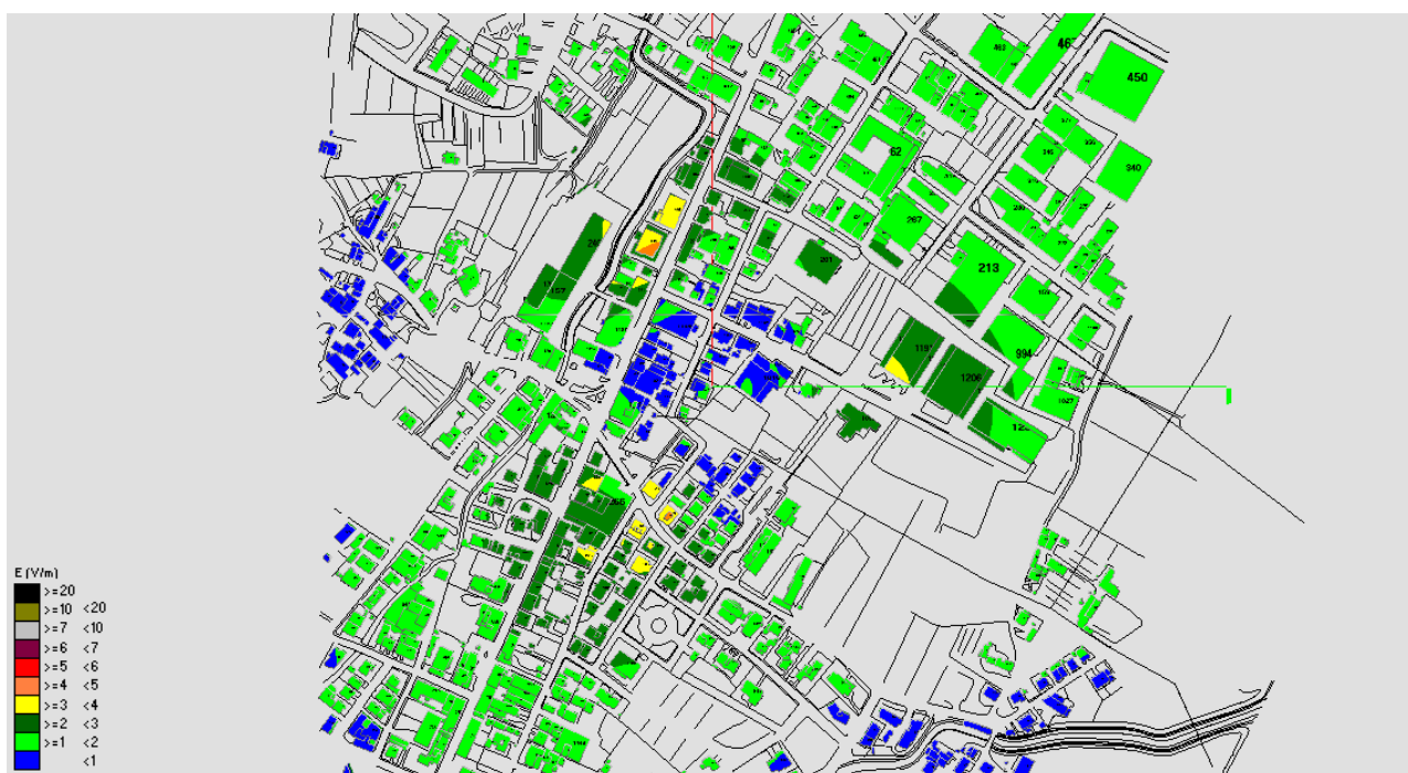
Fig. 14 Impatto elettromagnetico – Zona Centrale TELECOM Via Tiziano – Vista dall'alto
