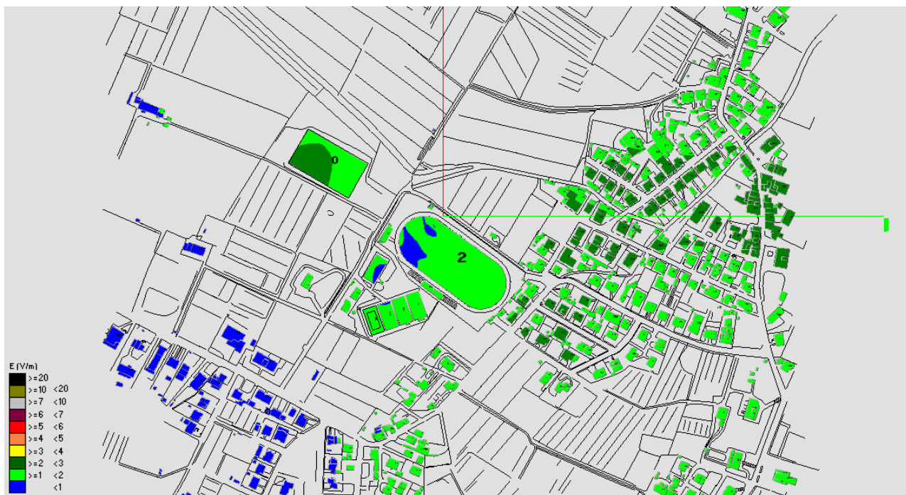
Fig. 20 Impatto elettromagnetico – Zona Stadio Comunale – Vista dall'alto
