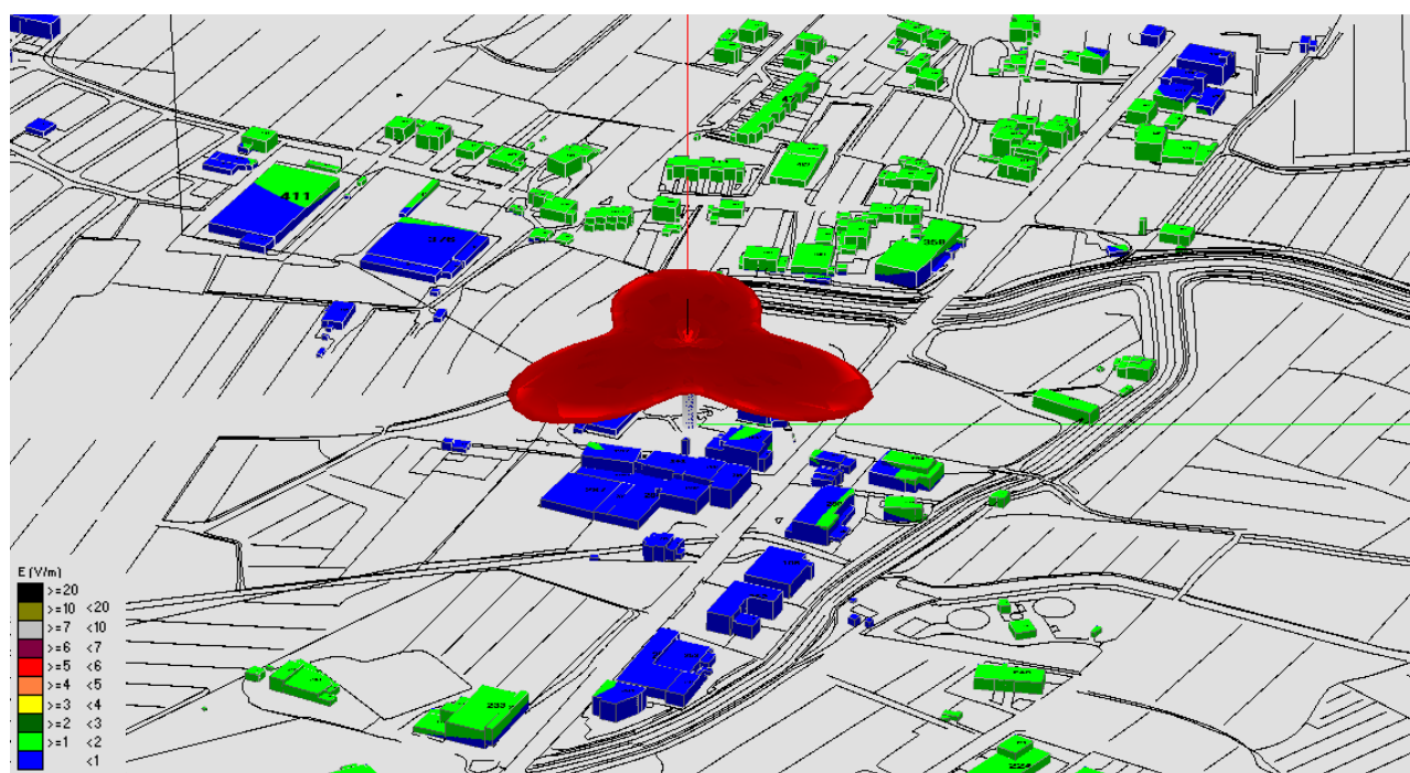
Fig. 7 Impatto elettromagnetico – Zona Torre Acquedotto – 0°/Nord
