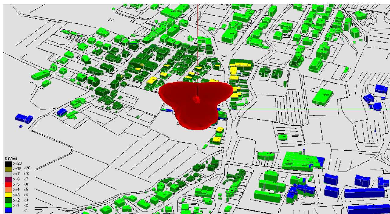
Fig. 22 Impatto elettromagnetico – Zona Via Mascagni – 0°/Nord
