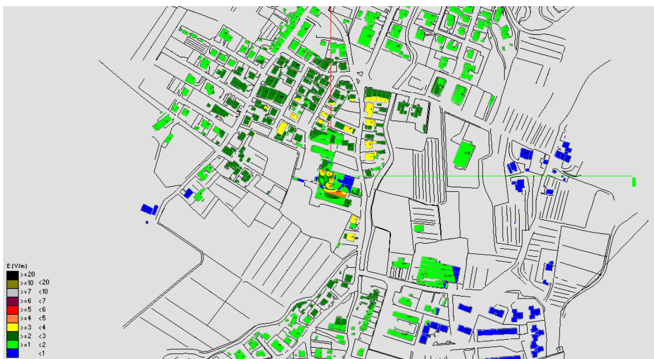
Fig. 23 Impatto elettromagnetico – Zona Via Mascagni – Vista dall'alto
