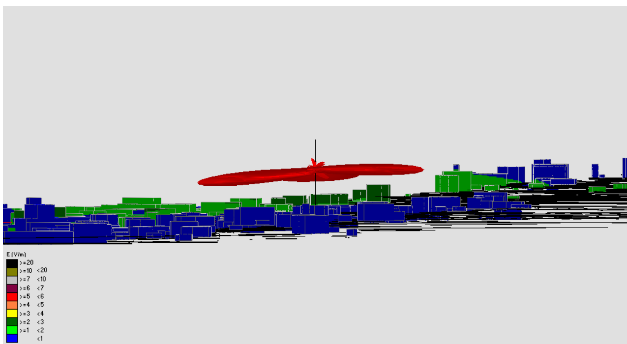
Fig. 6 Impatto elettromagnetico – Zona Cimitero Valenzatico – Vista Laterale
