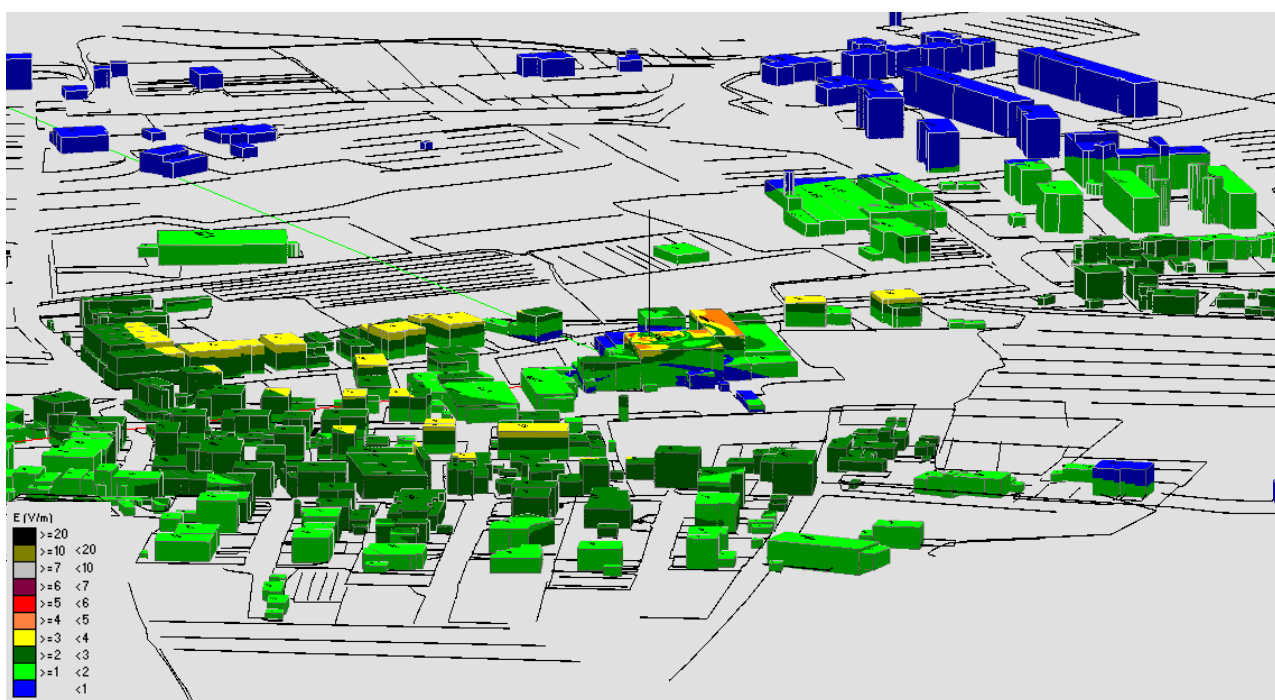
Fig. 24 Impatto elettromagnetico – Zona Via Mascagni – Vista Laterale
